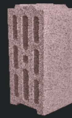
DDB - 19 ÜÇ SIRA BOŞLUKLU 9 GÖZLÜ GEÇMELİ DUVAR BLOĞU
