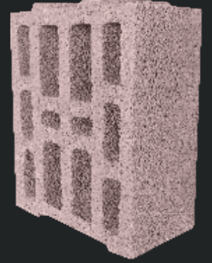
DDB - 30 DÖRT SIRA BOŞLUKLU 12 GÖZLÜ GEÇMELİ DUVAR BLOĞU
