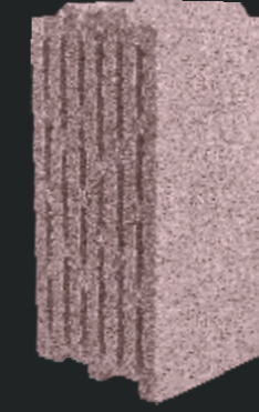
DDB - 19 SW ALTI SIRA BOŞLUKLU 21 GÖZLÜ GEÇMELİ DUVAR BLOĞU
